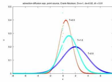
1+1 D Advection-Diffusion
